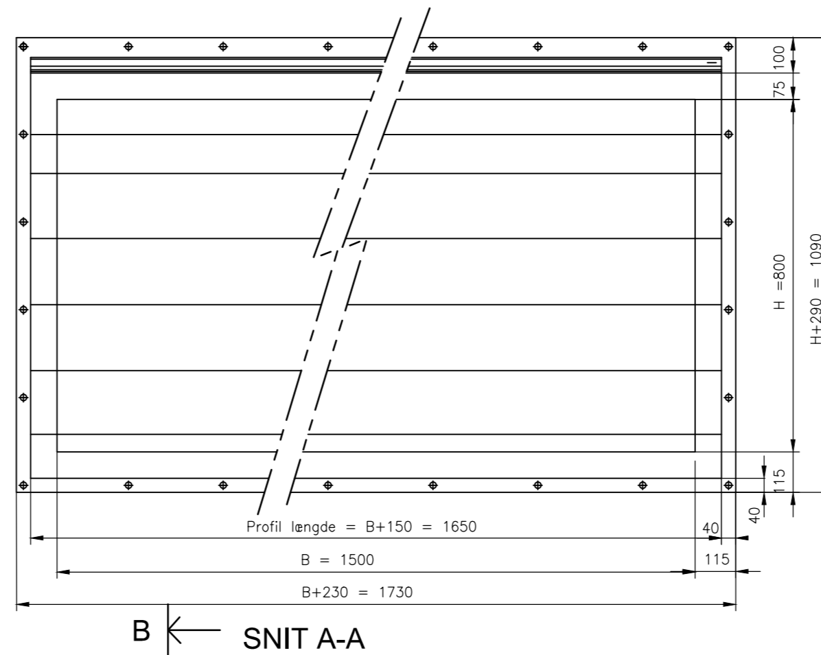
Kontraklap
