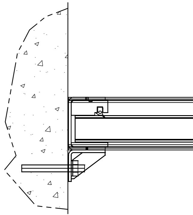
FASTGØRELSESDETALJE
