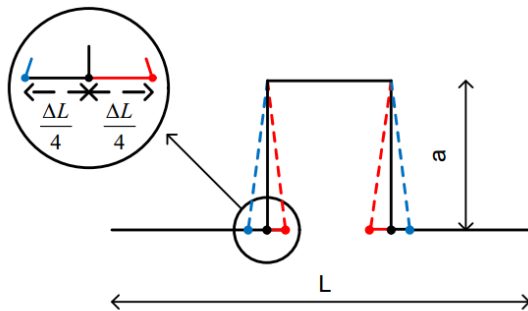
Figur 8 Ekspansionsarm ved lyre med forspænding
