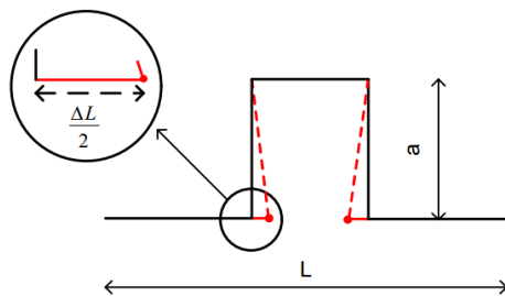
Figur 7 Ekspansionsarm ved lyre uden forspænding
