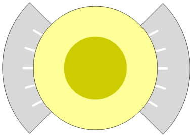
Figur 5 Tværsnit af præisoleret rør med skumpuder
