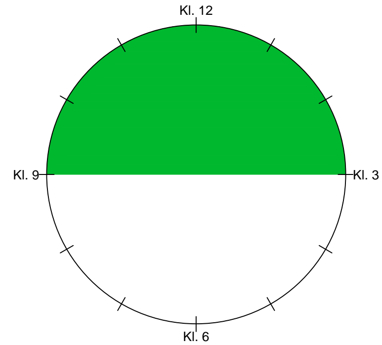
Placering af trækrør i ledningstværsnit over ø800mm
